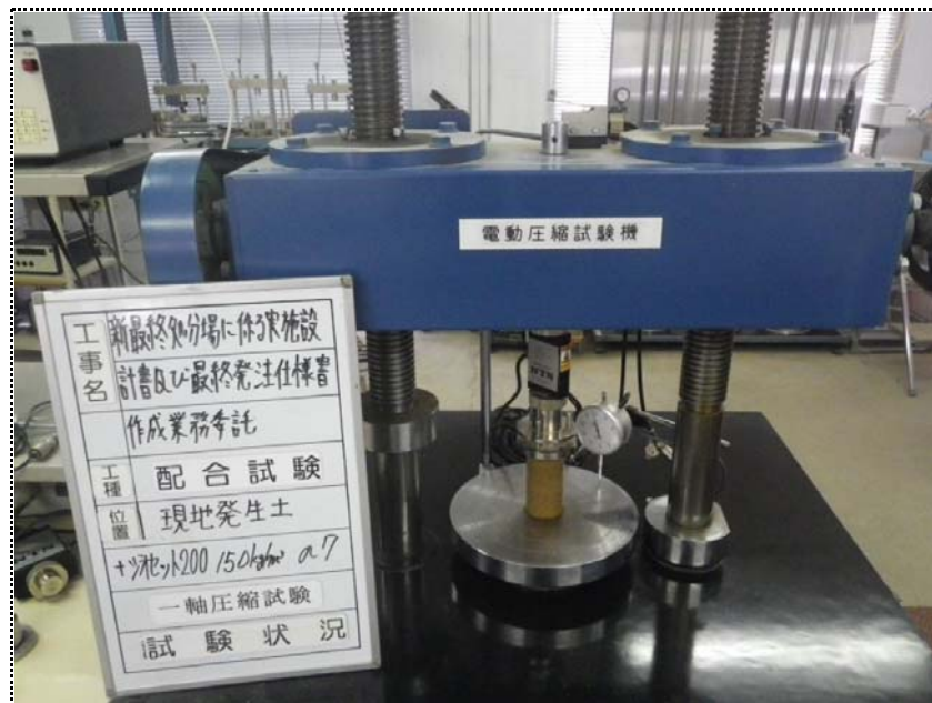
一軸圧縮試験 (試験状況) 150kg/m 3 (材令7日)
