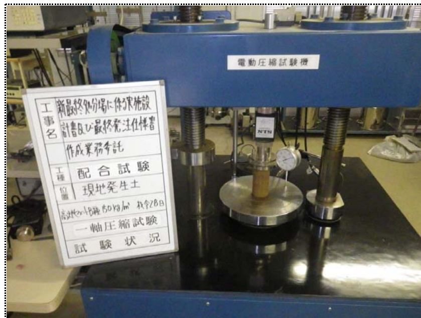
一軸圧縮試験（試験状況） 150kg/m³（材令28日）
