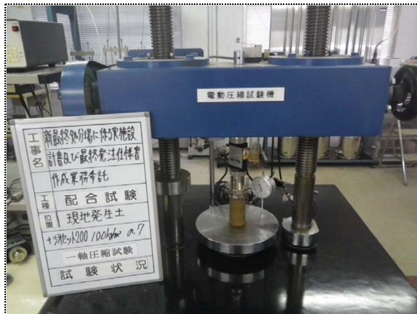
一軸圧縮試験 (試験状況) 100kg/m 3 (材令7日)
