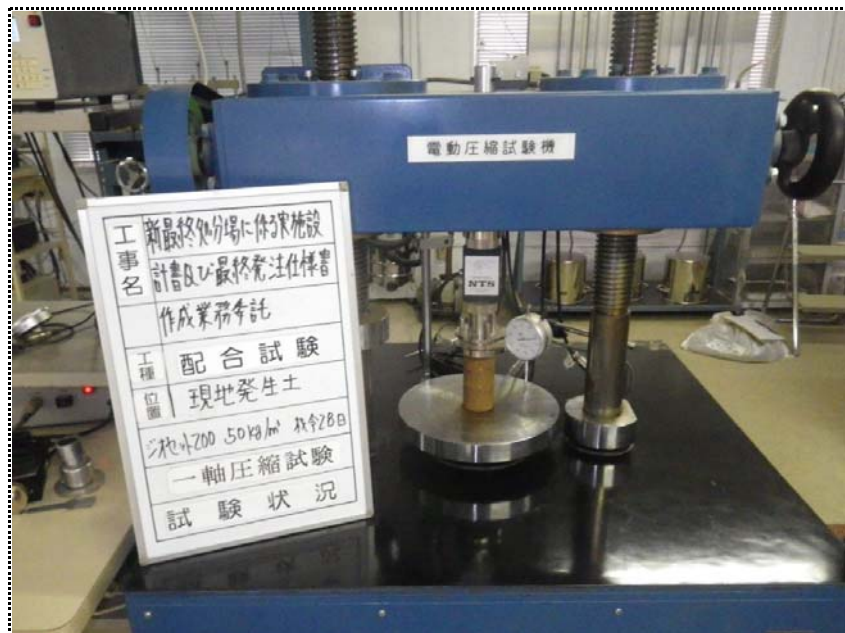
一軸圧縮試験 (試験状況) 50kg/m³ (材令28日)
