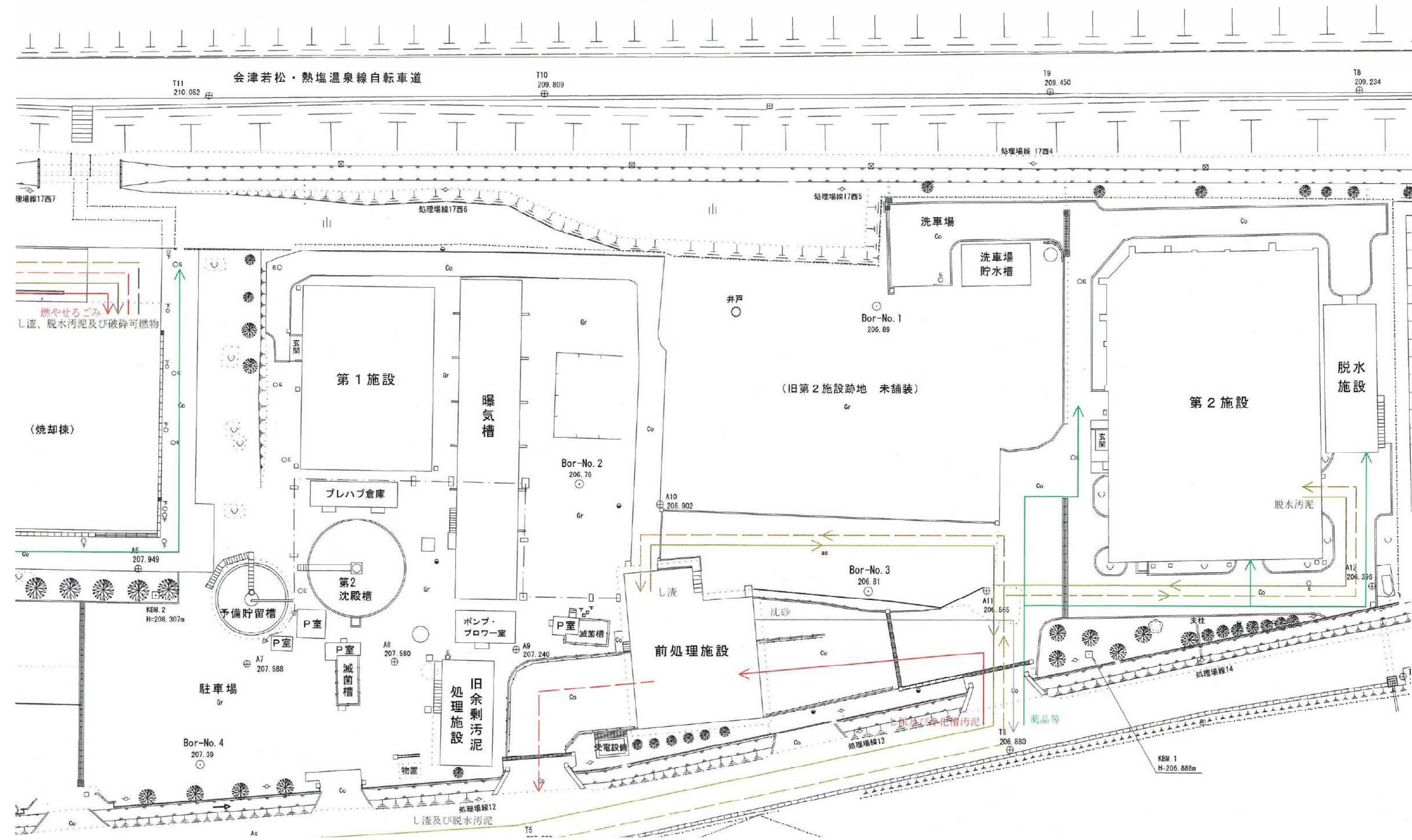
添付資料 28 関係車両動線図
