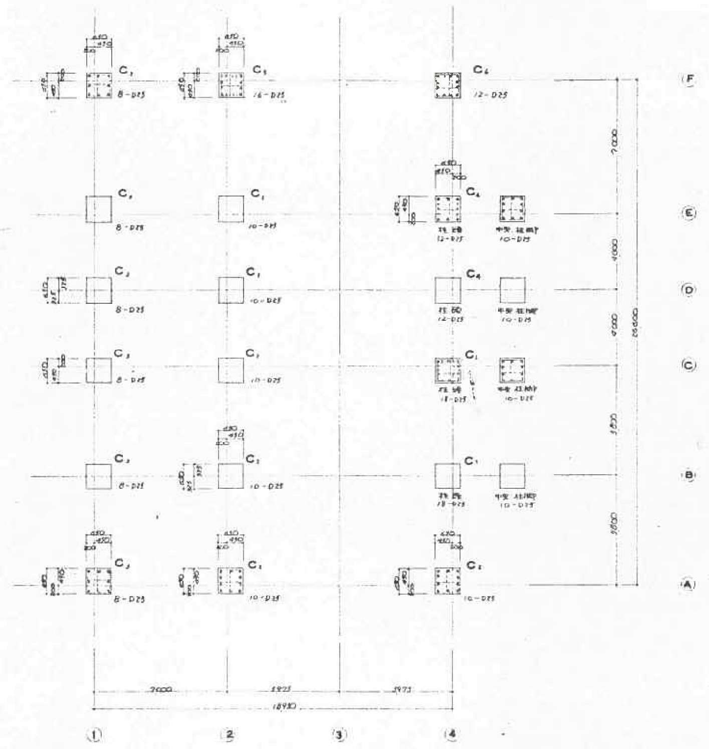
1 1E 2 1E 柱 伏図 - 単位 1/50
