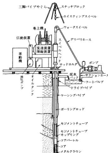
図3. 1-1 ハイドロリックフィード型ボーリング装置一般図
