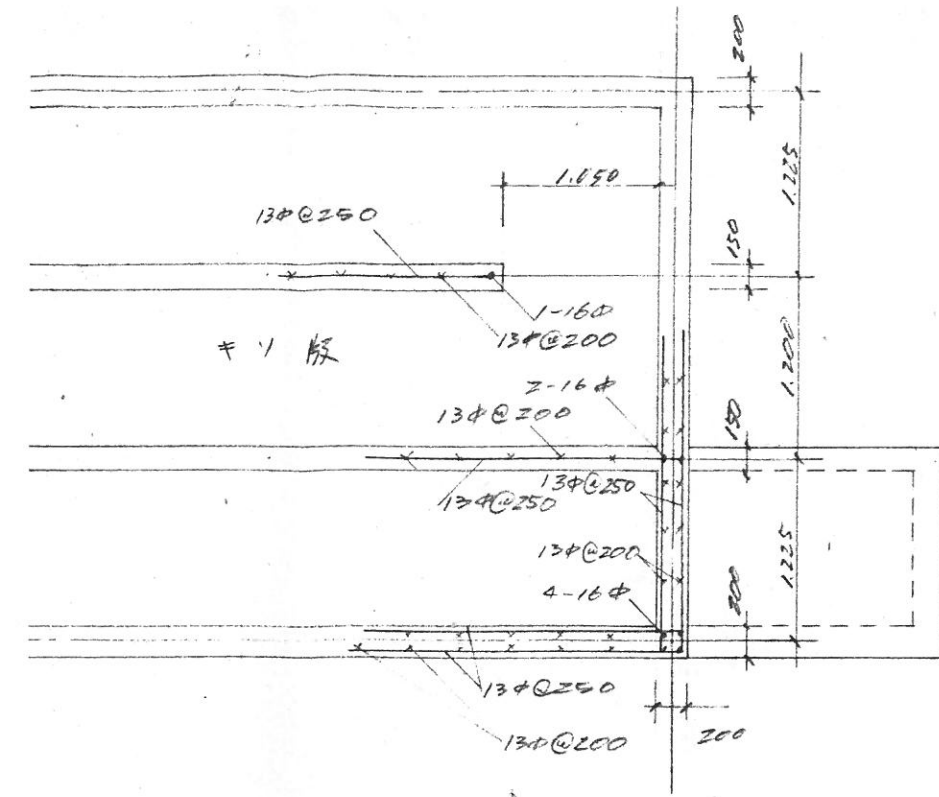
床版 1/50
