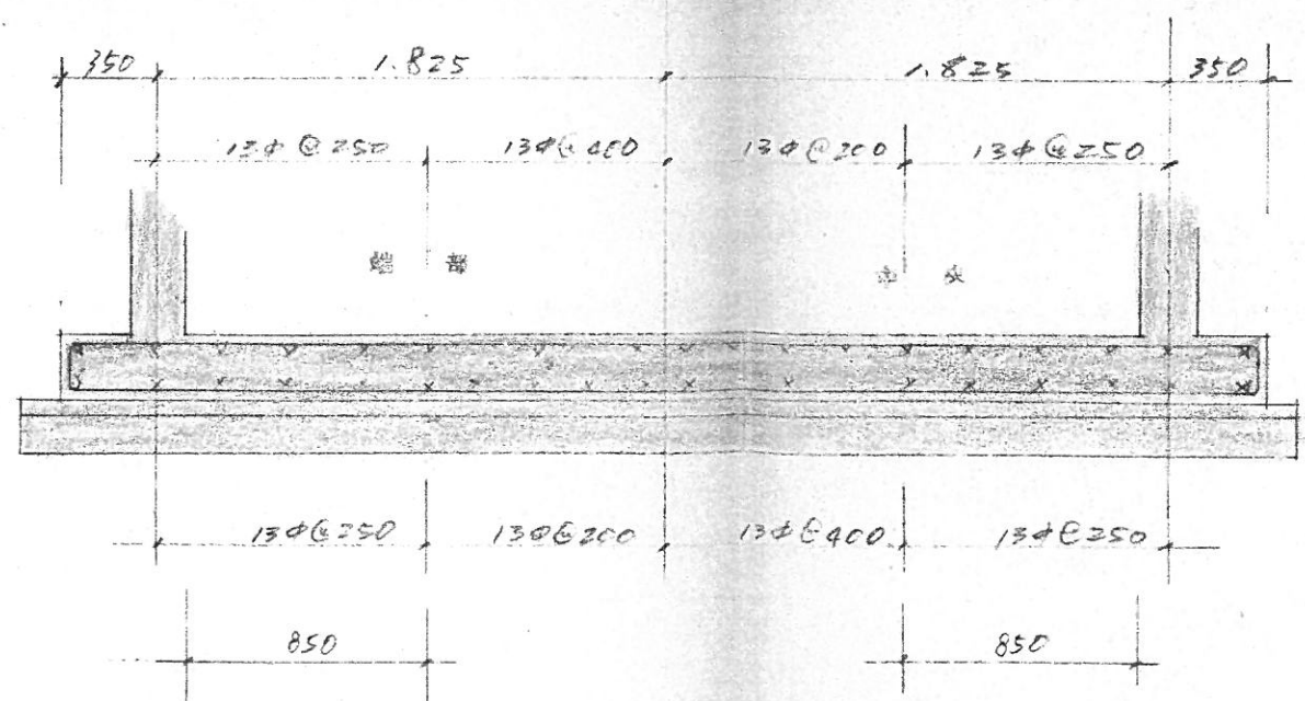
基礎版 1/30
