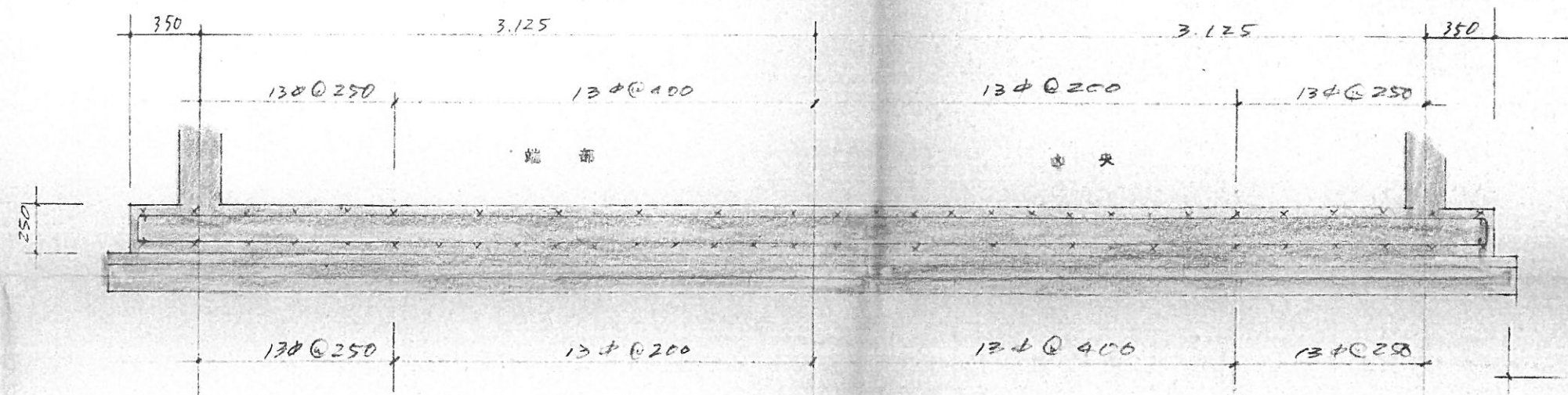
底口型 1/30
